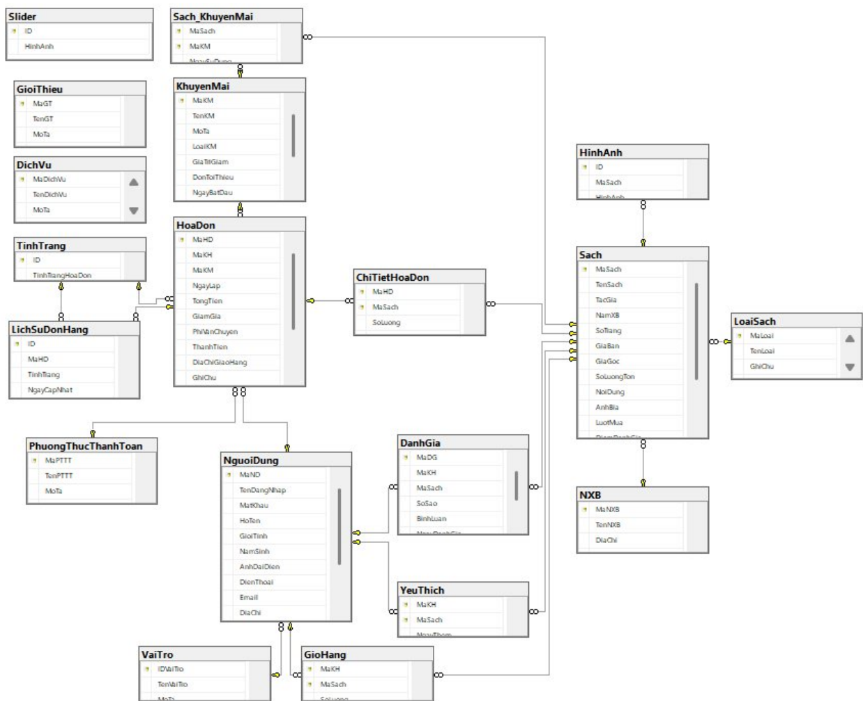
Hình 14-1 Sơ đồ thực thể - quan hệ (ERD)
